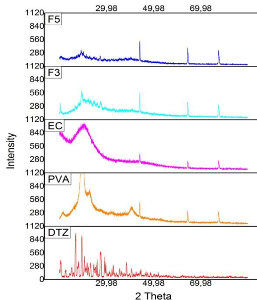
Gambar 3. Hasil uji difraksi sinar X diltiazem HCl murni, PVA, EC, serta film transdermal F3 dan F5
