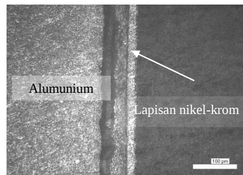
Gambar 2. Penampang melintang lapisan nikel pada aluminium dengan waktu pencelupan selama 30 menit
