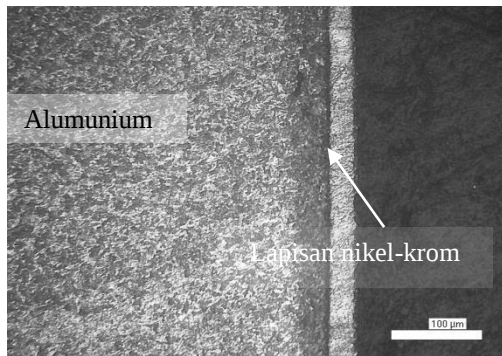
Gambar 4. Penampang melintang lapisan nikel pada aluminium dengan waktu pencelupan selama 60 menit
