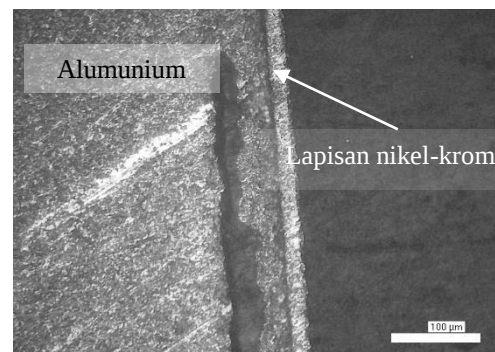
Gambar 3. Penampang melintang lapisan nikel pada aluminium dengan waktu pencelupan selama 45 menit
