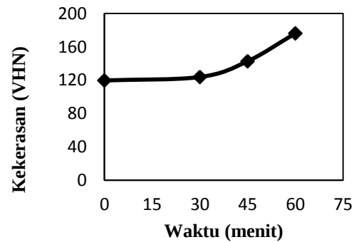
Gambar 6. Grafik hubungan kekerasan dan waktu pencelupan
