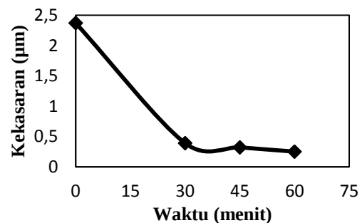
Gambar 7. Grafik hubungan kekasaran dan waktu pencelupan
