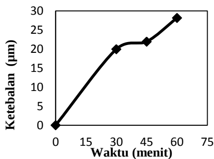
Gambar 5. Grafik hubungan ketebalan lapisan nikel terhadap lama waktu pencelupan
