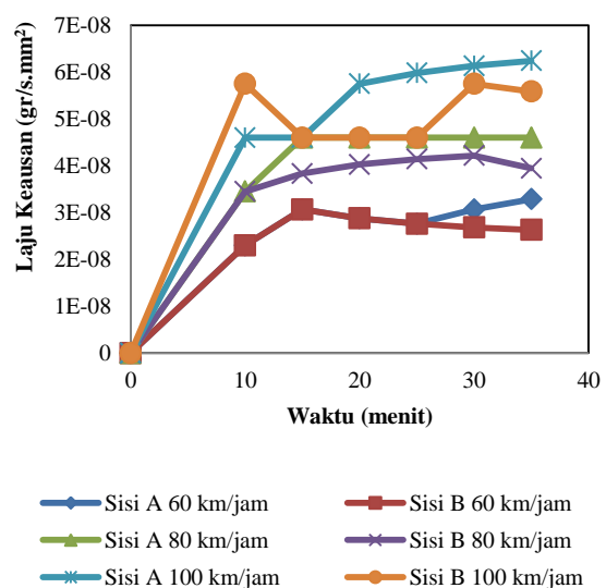
Gambar 7 Grafik laju keausan sisi kampas A dan sisi kampas B pada masing-masing kecepatan
