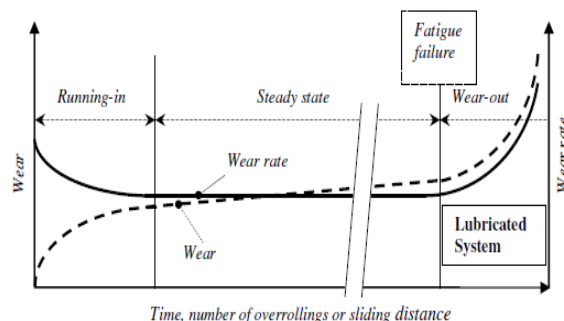
Gambar 1 Grafik tahapan keausan (Jamari, 2006)
