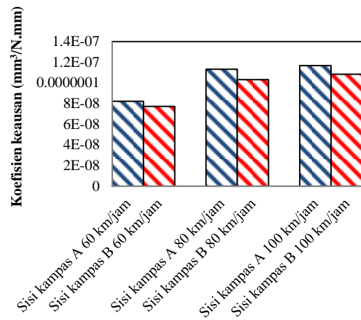
Gambar 6 Koefisien Keausan yang terjadi pada sisi kampas A dan sisi kampas B pada masing-masing kecepatan
