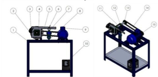
Gambar 3 Gambar teknik alat uji keausan kampas rem
