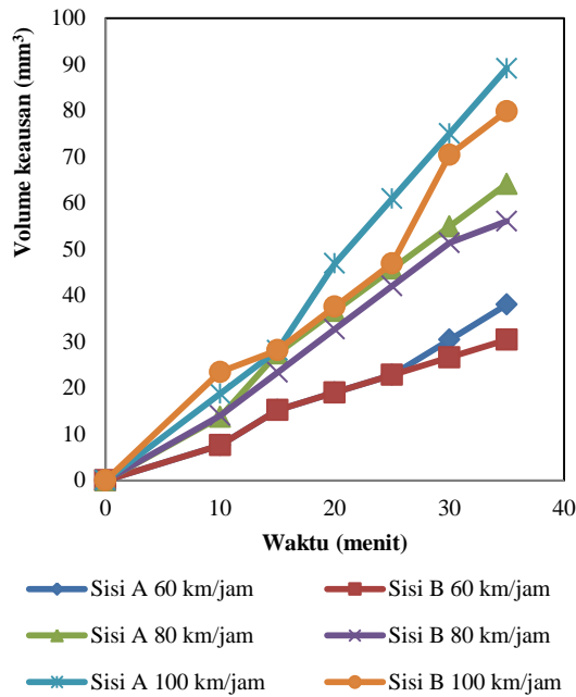
Gambar 5 Grafik hubungan volume keausan dengan waktu pada sisi kampas A dan sisi kampas B pada masing-masing kecepatan
