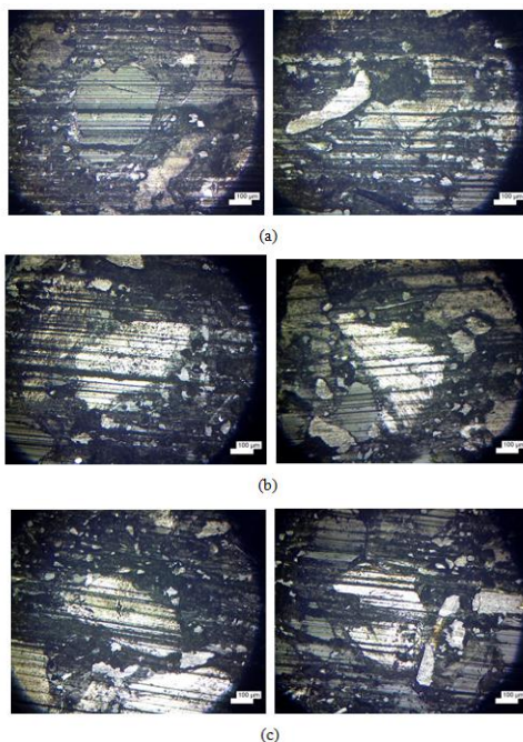
Gambar 8 Hasil foto mikro waktu pengujian 35 menit sisi kampas A dan B dengan perbesaran 100 kali untuk variasi kecepatan (a) 60 km/jam, (b) 80 km/jam, (c) 100 km/jam.
