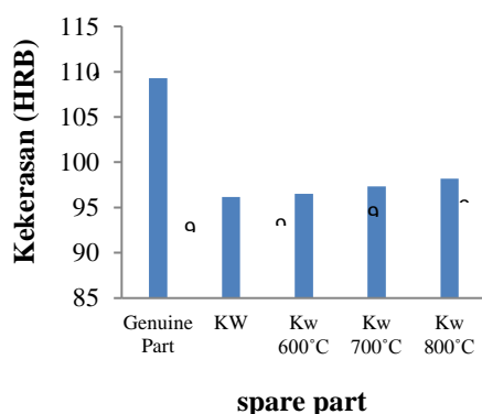
Gambar 1. Hasil uji kekerasan (HRB)
