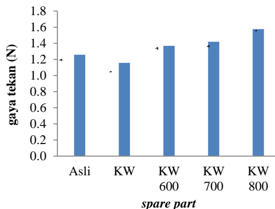
Gambar 10. Grafik gaya tekan ring piston
