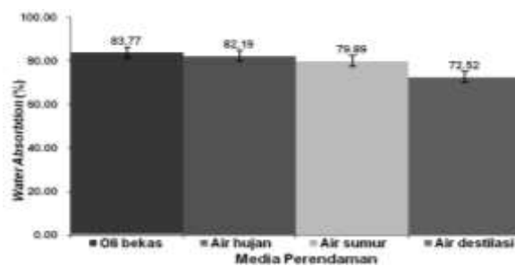
Gambar 1. Pengaruh media perendaman terhadap water absorption
