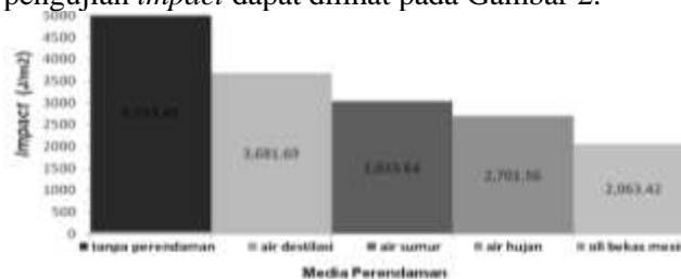
Gambar 2. Pengaruh media perendaman terhadap kekuatan impact
