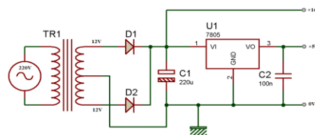
Gambar 5. Rangkaian Catu Daya
