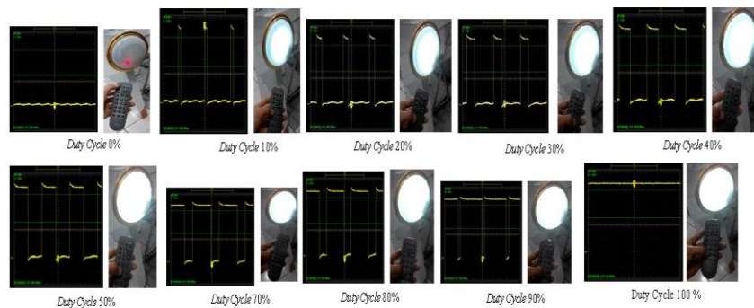
Gambar 9. Testing Lampu LED dengan Sinyal PWM
