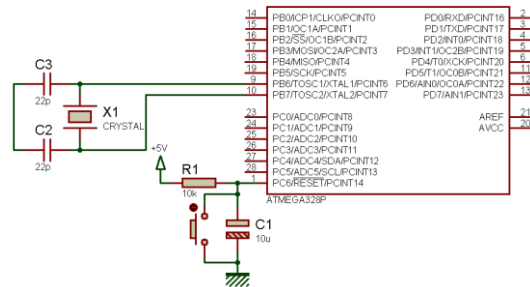
Gambar 2. Rangkaian Sistem Minimum Microcontroller ATmega328
