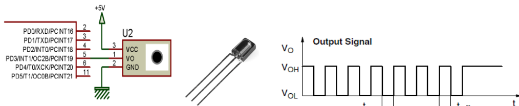
Gambar 3. Rangkaian Interface, Fisik Sensor, dan Bentuk Sinyal Output TSOP38238
