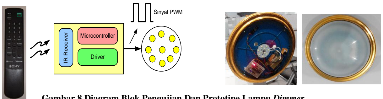
Gambar 8 Diagram Blok Pengujian Dan Prototipe Lampu Dimmer
