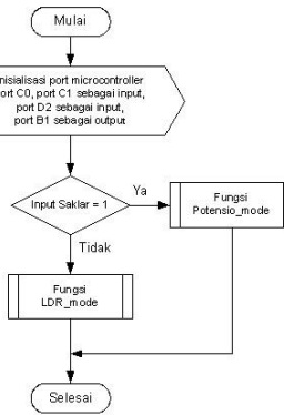
Gambar 6. Diagram Alir Perangkat Lunak Pengendali Lampu Dimmer LED
