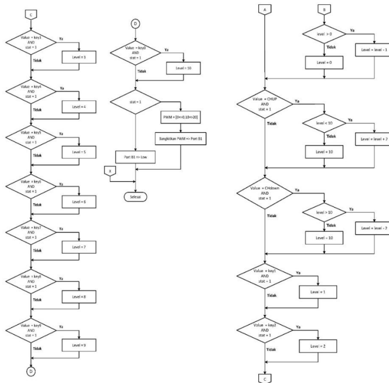
Gambar 7. Subprogram Sistem
