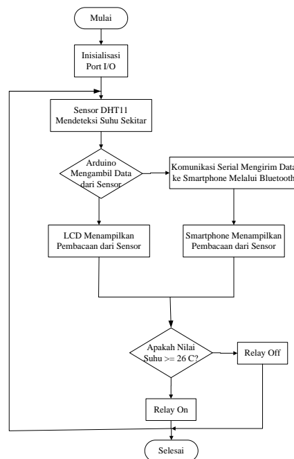
Gambar 2. Flowchart Cara Kerja Sistem Pendingin Perangkat Telekomunikasi
