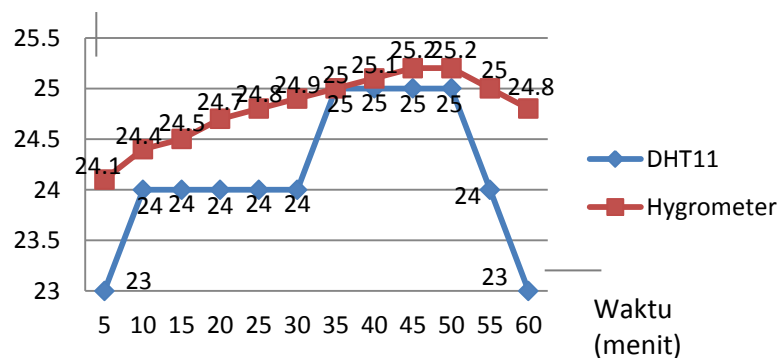
Gambar 3. Grafik Perbandingan Hasil Pengujian Sensor DHT11 dan Thermohygrometer .
