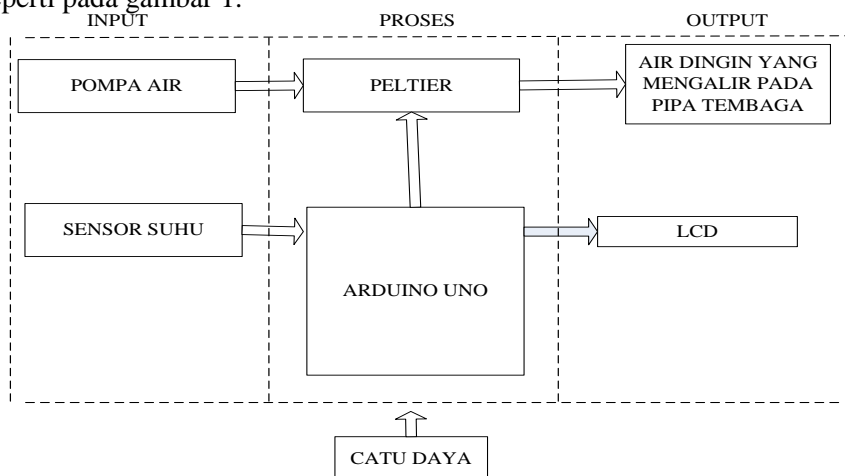
Gambar 1. Blok Diagram Sistem
