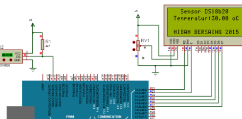
Gambar 15. Simulasi Rangkaian Sensor DS18B20 Menggunakan
