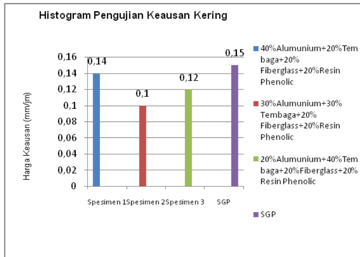
Gambar 1. Histogram Hasil Pengujian Keausan kering
