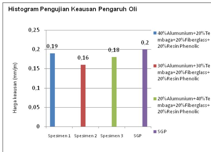
Gambar 2. Histogram Hasil uji Keausan Pengaruh Oli
