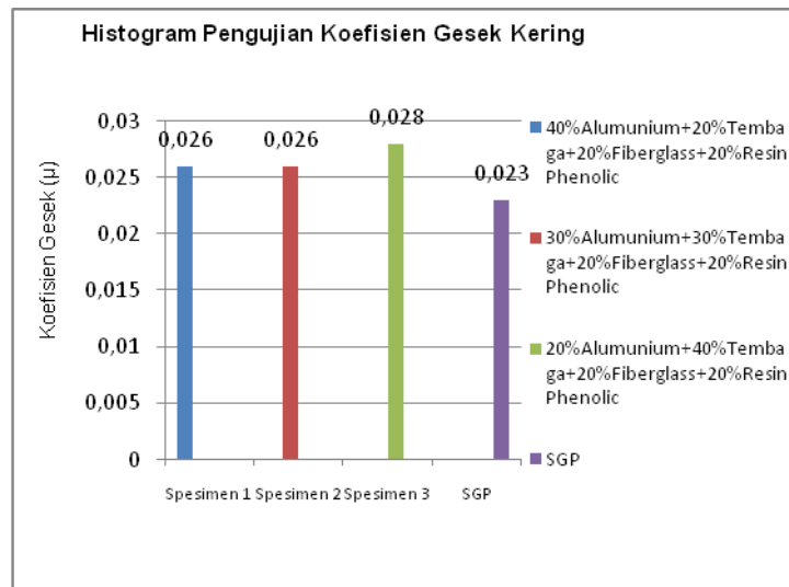
Gambar 3. Histogram Hasil koefisien gesek kering
