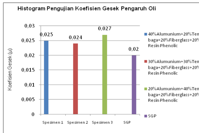
Gambar 4. Histogram Hasil koefisien gesek oli
