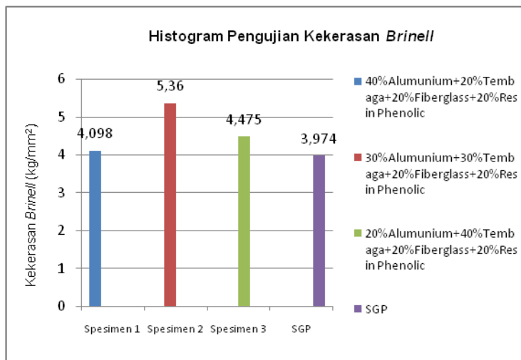
Gambar 5. Histogram Hasil uji kekerasan
