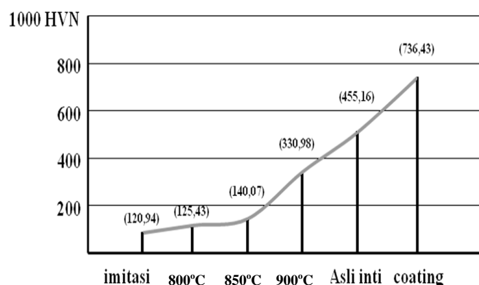
Gambar 6. Grafik Kekerasan sproket Supra 125 sebelum dan sesudah di heat treatment
