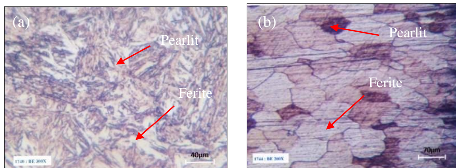
Gambar 3 Foto Strukturmikro sproket (a) asli (b) Imitasi
