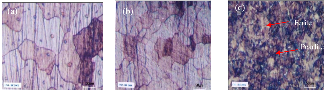
Gambar 4. Foto Strukturmikro karburizing (a) 800°C (b) 850°C (c) 900°C
