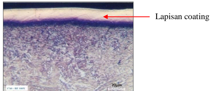
Gambar 5. Foto Struktur Mikro lapisan coating .
